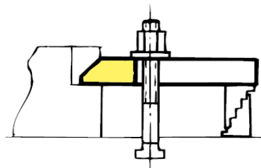
Vidlicová upínka s nosem; DIN 6315 GN, materiál zušlechtěná ocel, lakovaná
